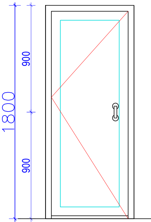
DOOR-D2 (4 Nos.)
