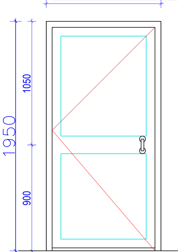
DOOR-D1 (4 Nos.)
